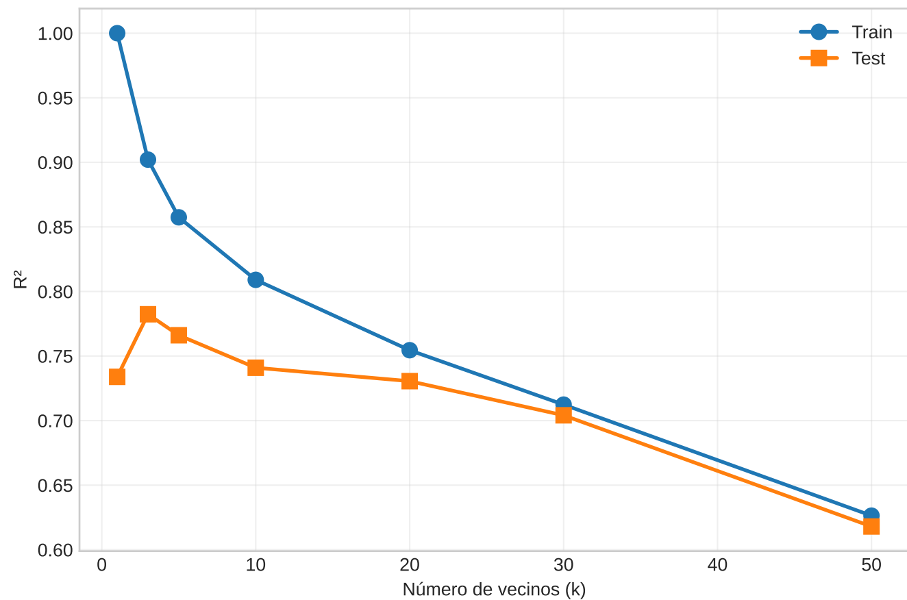
R 2 vs k en KNN
