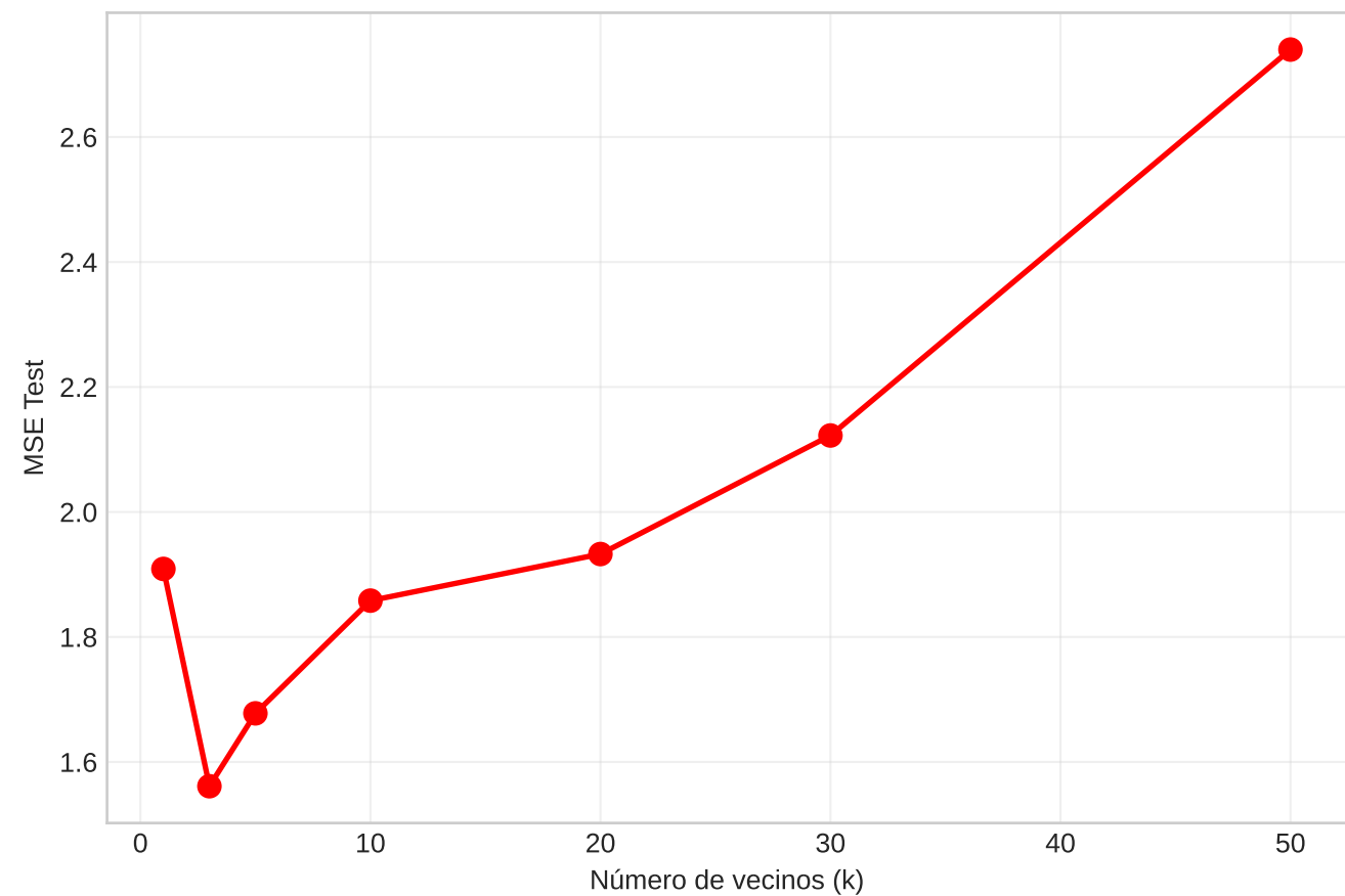
MSE vs k en KNN
