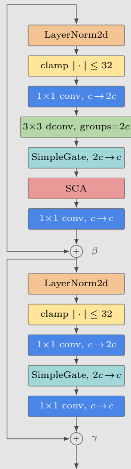
(d) enc3 block c = 128 , 8 blocks
