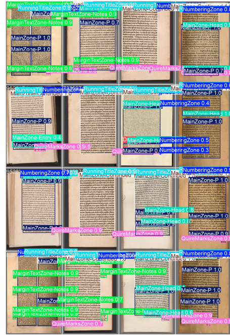
FIGURE 3 – Prédiction effectuées par notre modèle.
