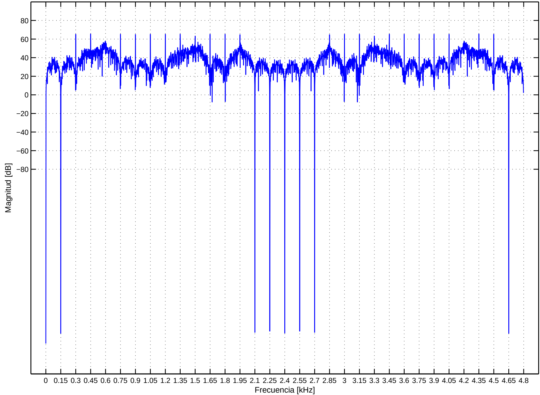
Espectro de la señal OFDM
