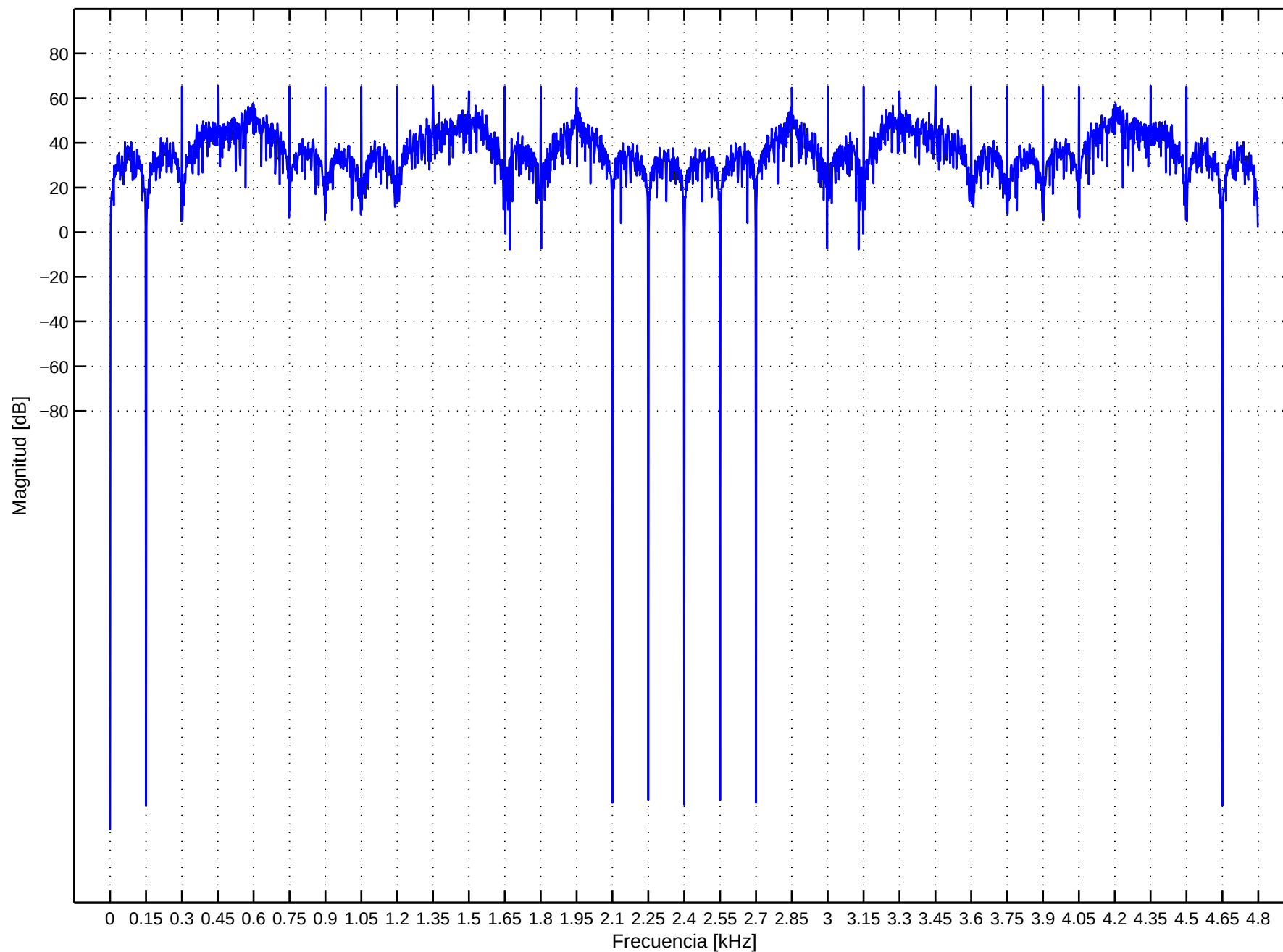
Espectro de la señal OFDM
