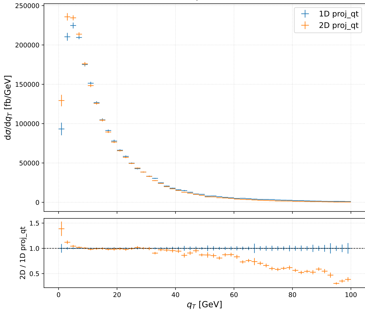
W^+ — NNLL, scala nominale
