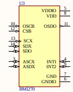
GNDIO
