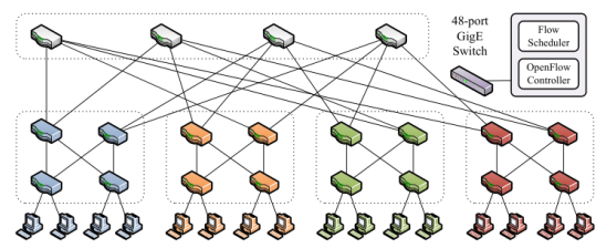
Flow Scheduler 统一调整数据平面路径
