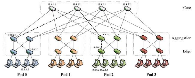
多级 Fat-Tree 提供跨 Pod 等价路径
