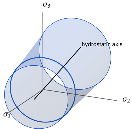
(a) von Mises cylinder
