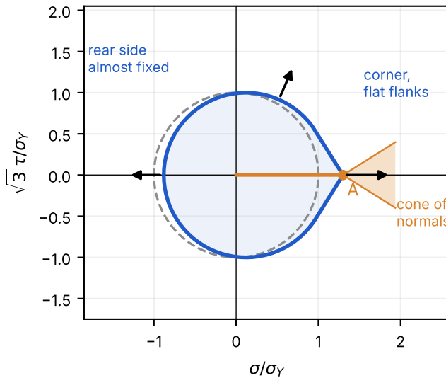
(d) distortion observed (schematic, after Bui)
