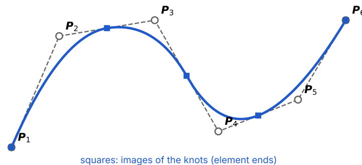
(d) quadratic B-spline curve and control polygon
