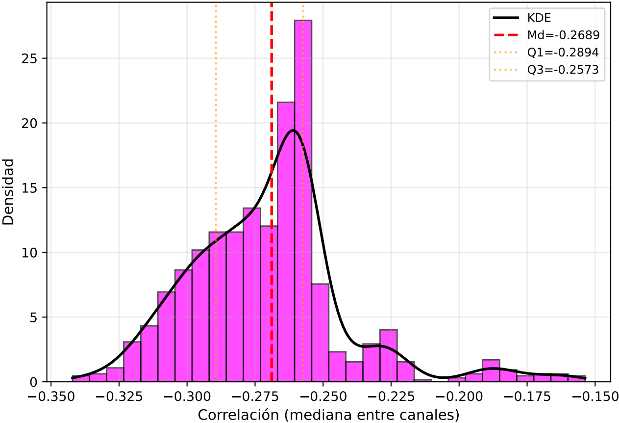
Histograma + KDE
