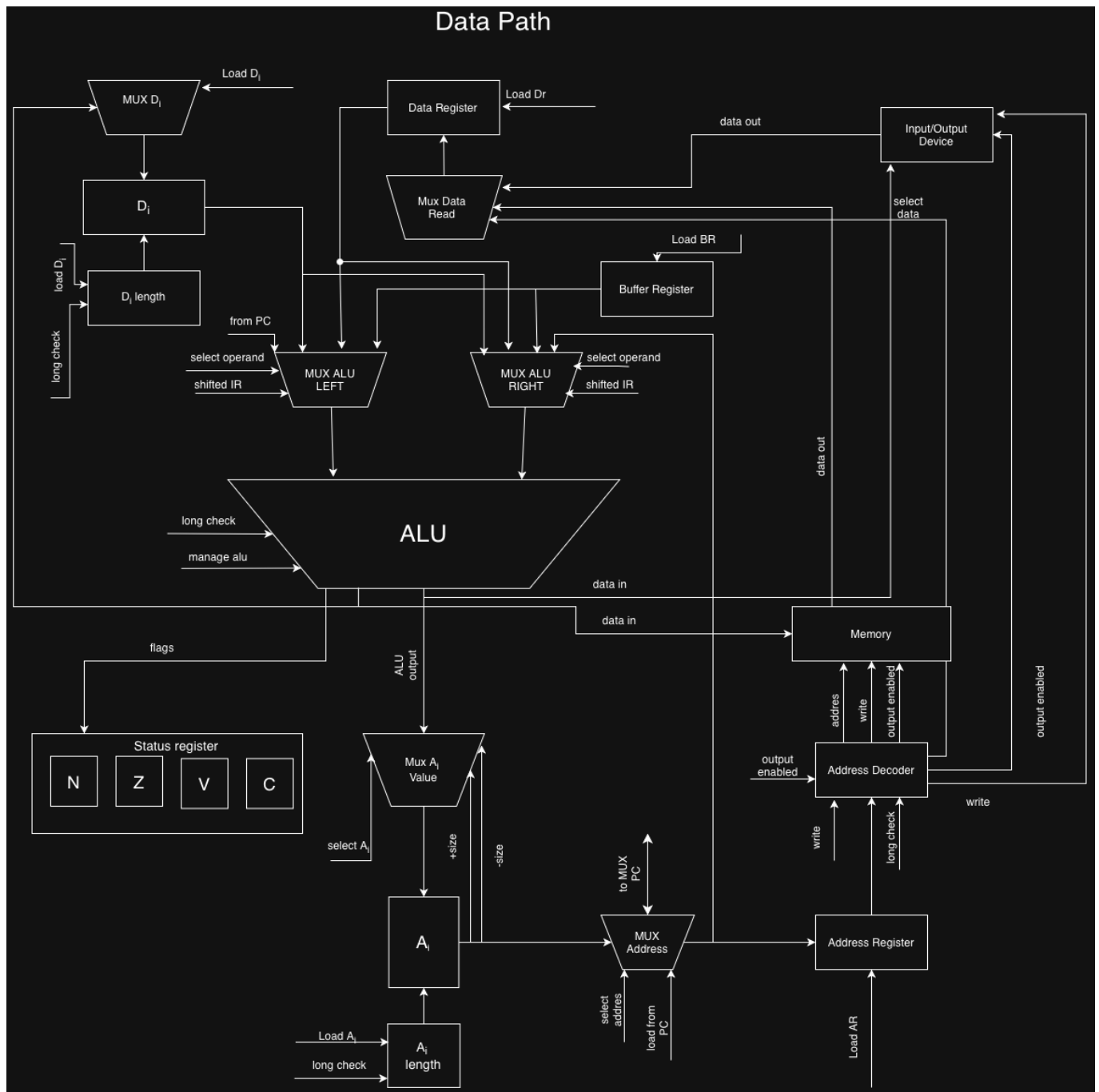
Рис. 2: Data Path
