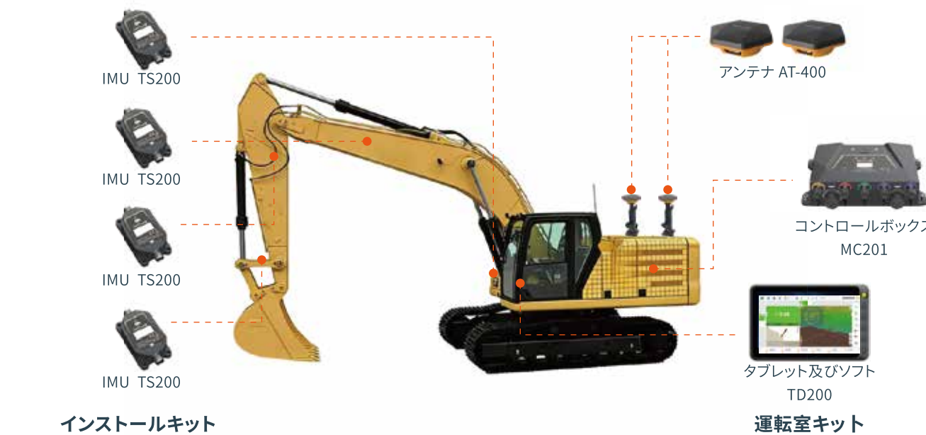
E50-Flexidig 3D
