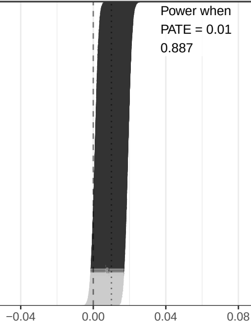
Simulated posterior estimate
