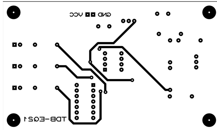
typon de la couche BOTTOM du circuit:
