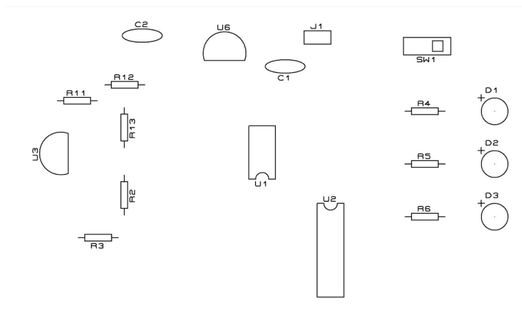
Schéma d'implantation du circuit
