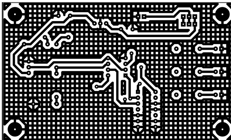
typon de la couche TOP du circuit:
