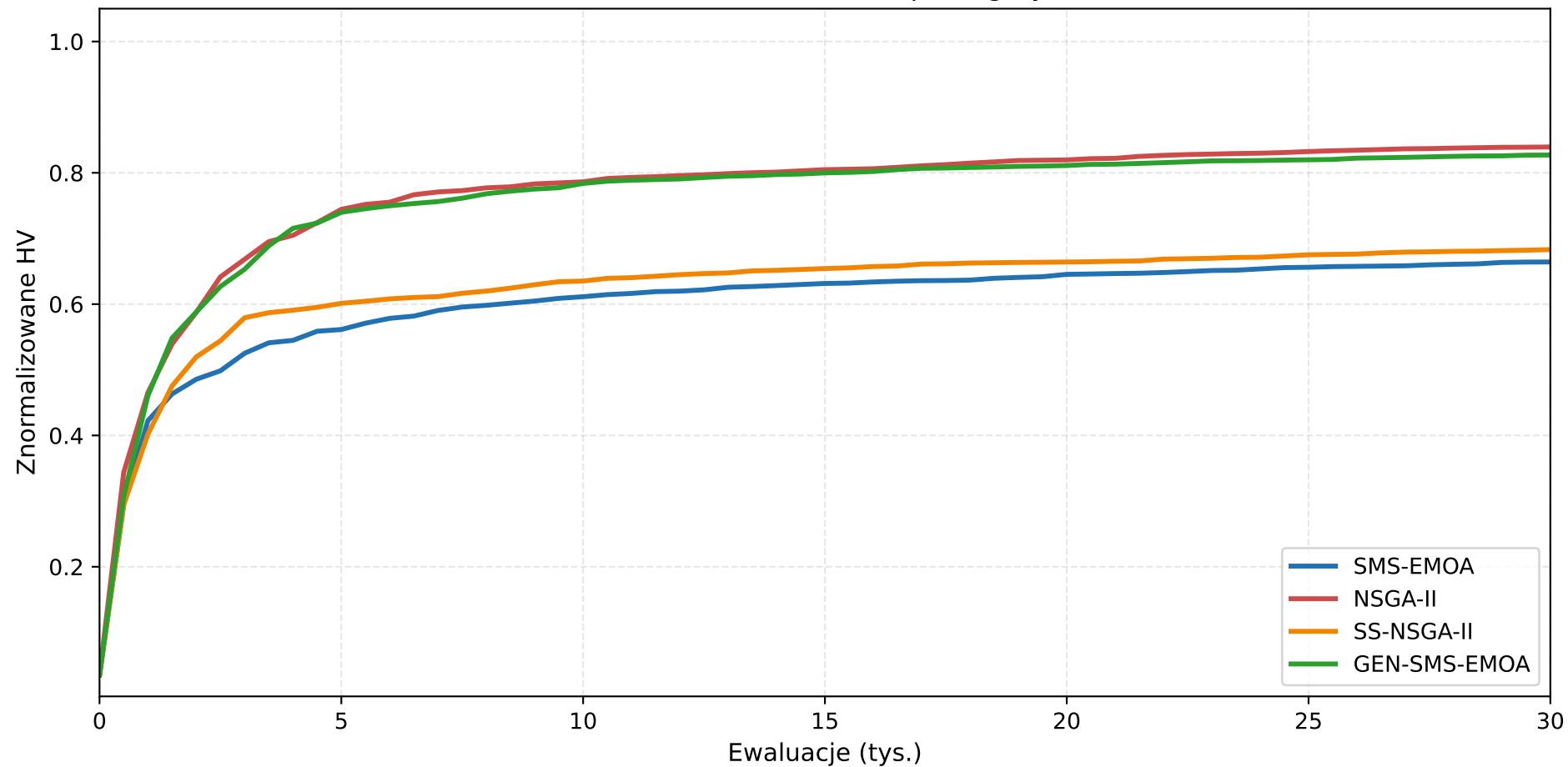
Konwergencja HV — instancja tcW mediana \pm IQR (30 ziaren per algorytm)
