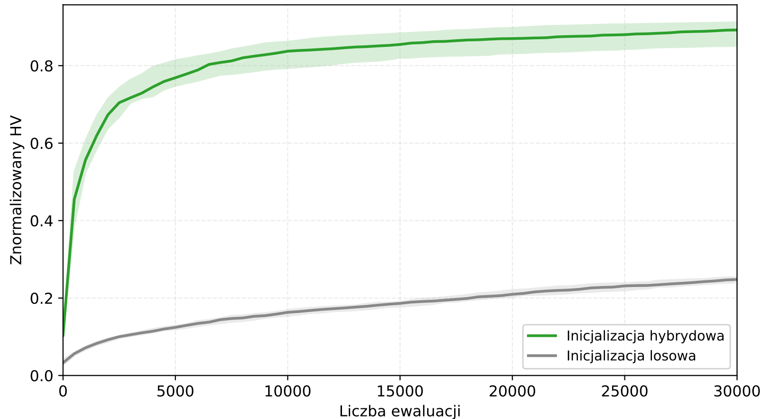
Konwergencja SMS-EMOA — inicjalizacja hybrydowa vs losowa instancja tcGB, mediana \pm IQR (30 ziaren)
