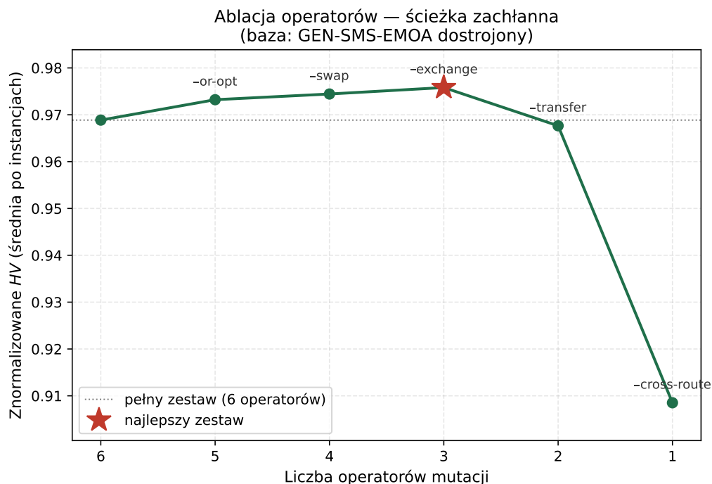
Rysunek 4.4. Ścieżka ablacji operatorów mutacji na dostrojonym wariantcie GEN-SMS-EMOA: znormalizowane HV (średnia po ośmiu instancjach) w miarę usuwania operatorów po jednym (od sześciu do jednego). Przy każdym punkcie podano usunięty operator; gwiazdka – najlepszy zestaw (trzy operatory).
