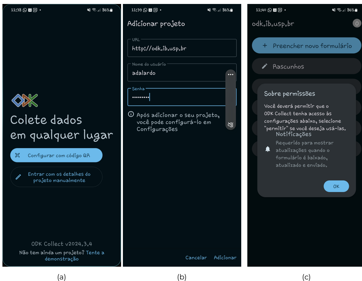
Figure 1.1: Criando conta manualmente no ODK Collect
