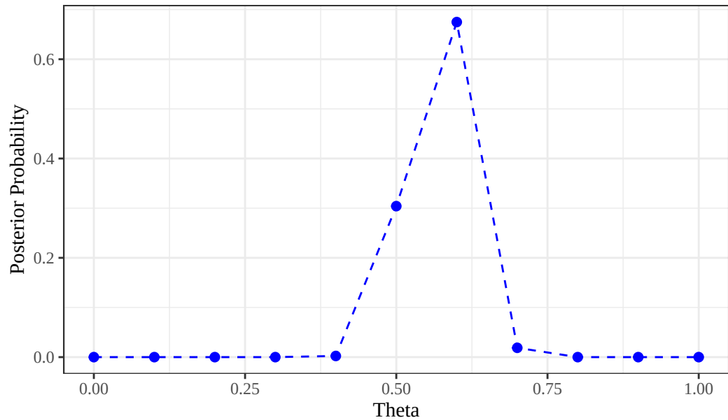
Posterior Probability Distribution P(. | Y = 57)
