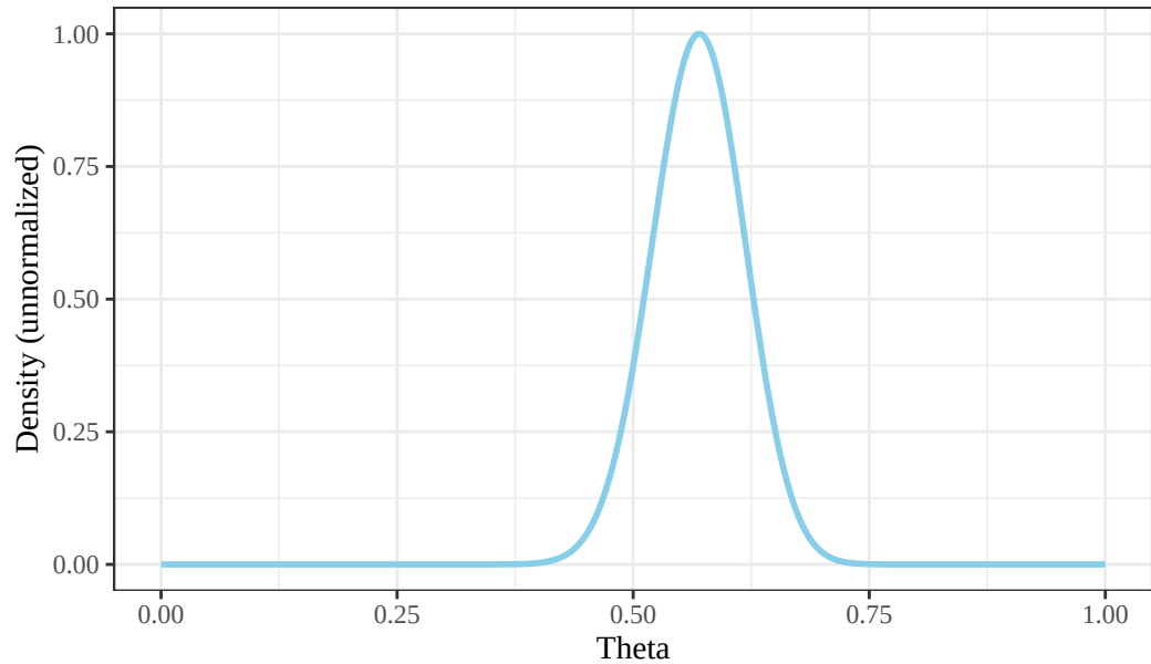
Posterior Density p(\cdot \mid Y = 57)
