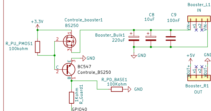
Circuit_commandement
