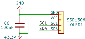
Circuit_Affichage
