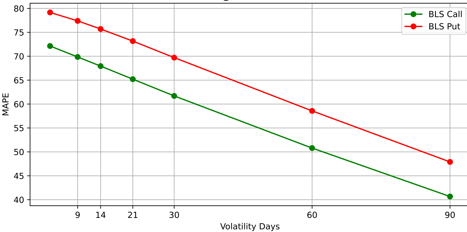
Testing — BLS MAPE
