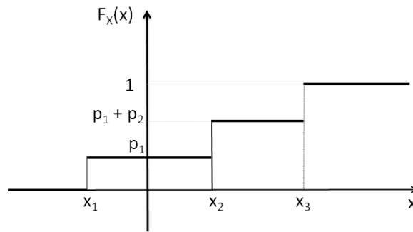
Figura 2.1: Funció de distribució d'una variable discreta.
