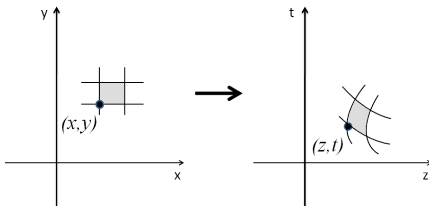
Figura 6.2: Canvi de l'element de mesura.
