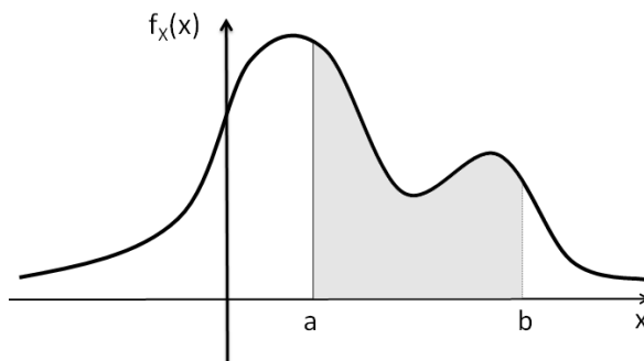
Figura 2.2: Probabilitat com àrea sota f_X . L'àrea ombrejada és igual a P(a \leq X \leq b) .
