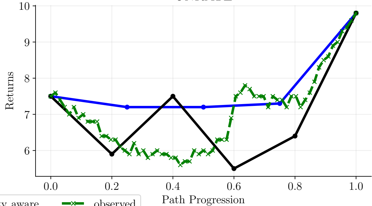
UNRATE
