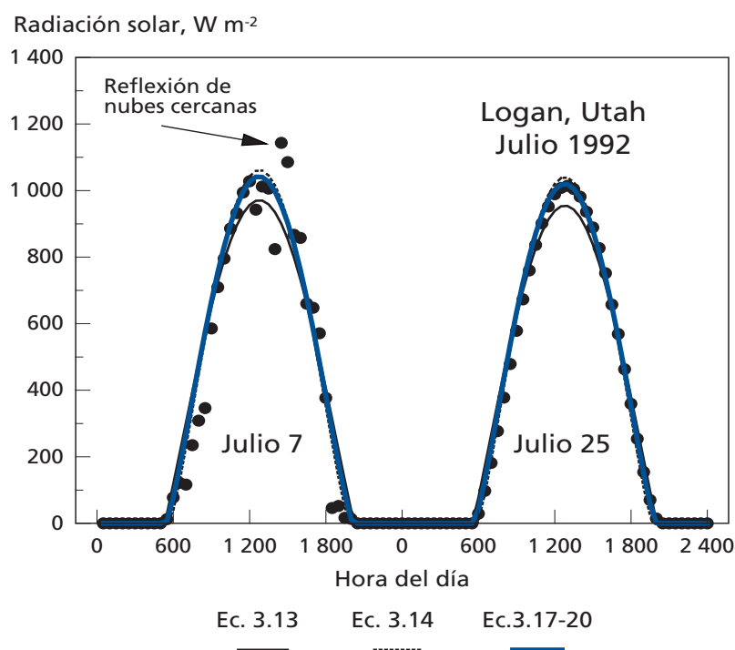
FIGURA A5.2 Promedios de lecturas de 30-minutos de R_s y de R_{so} estimada en Logan, Utah el 7 y el 25 de Julio de 1992
