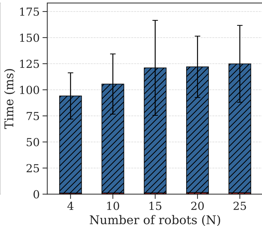
SECaaS (Verifier)
