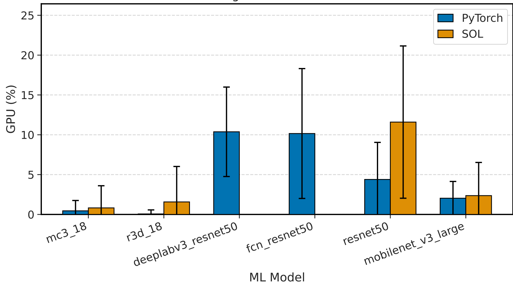
Edge GPU utilization
