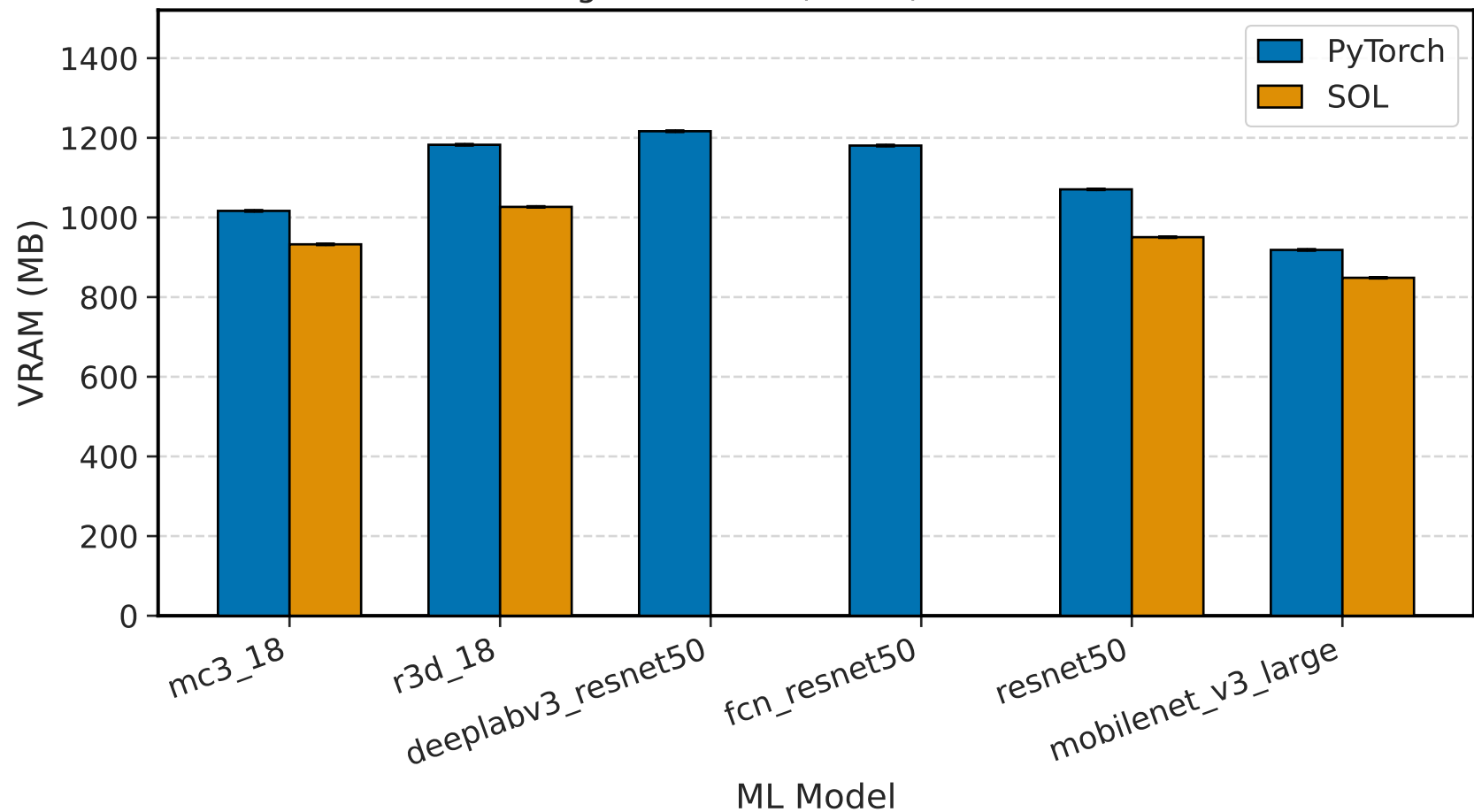
Edge GPU RAM (VRAM) utilization
