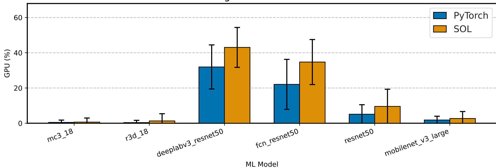
Edge GPU utilization
