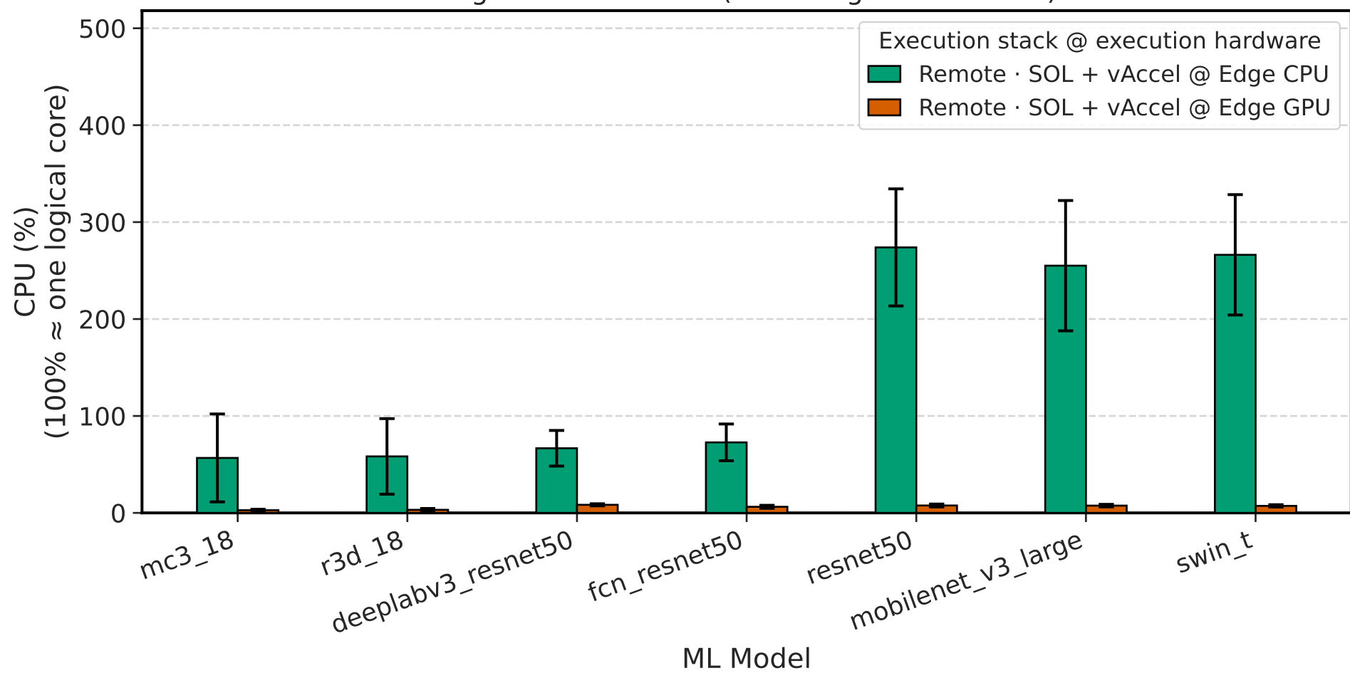
Edge CPU utilization (vaccel-agent container)
