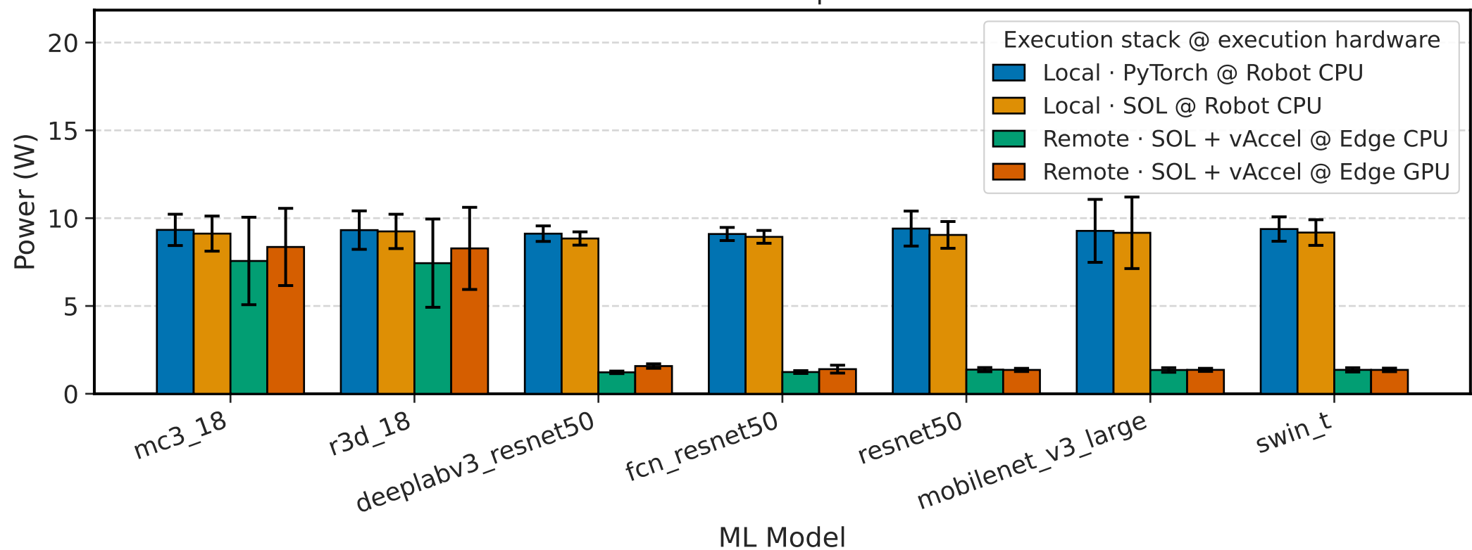
Edge CPU power
