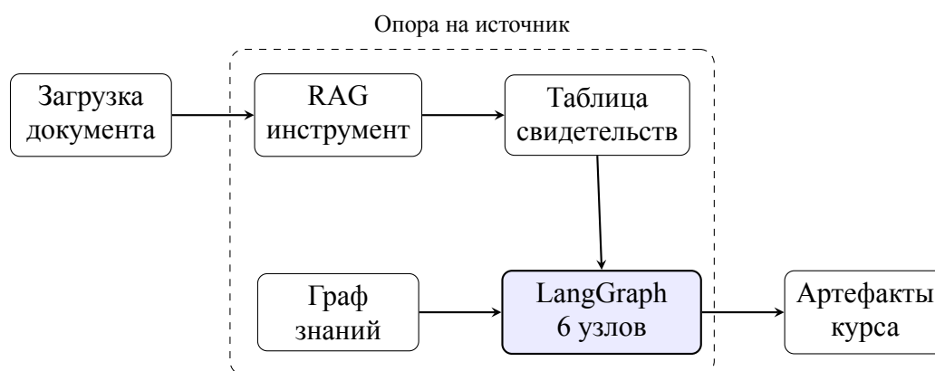
Рисунок 2.1 — Технологический стек ИИ-методиста: опора на источник и генерация
