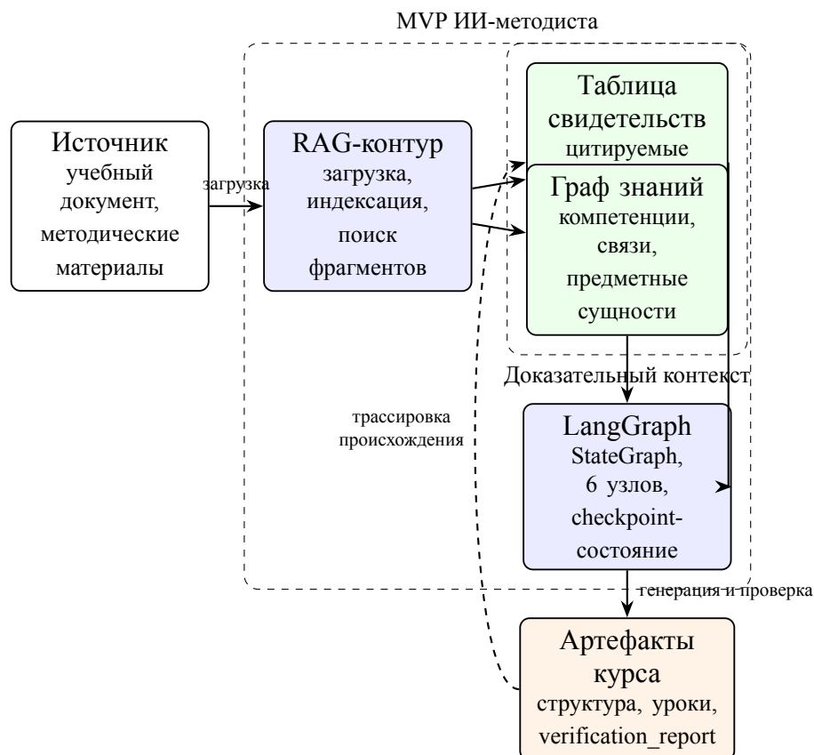
Рисунок 2.1 — Компонентная схема текущего MVP ИИ-методиста
