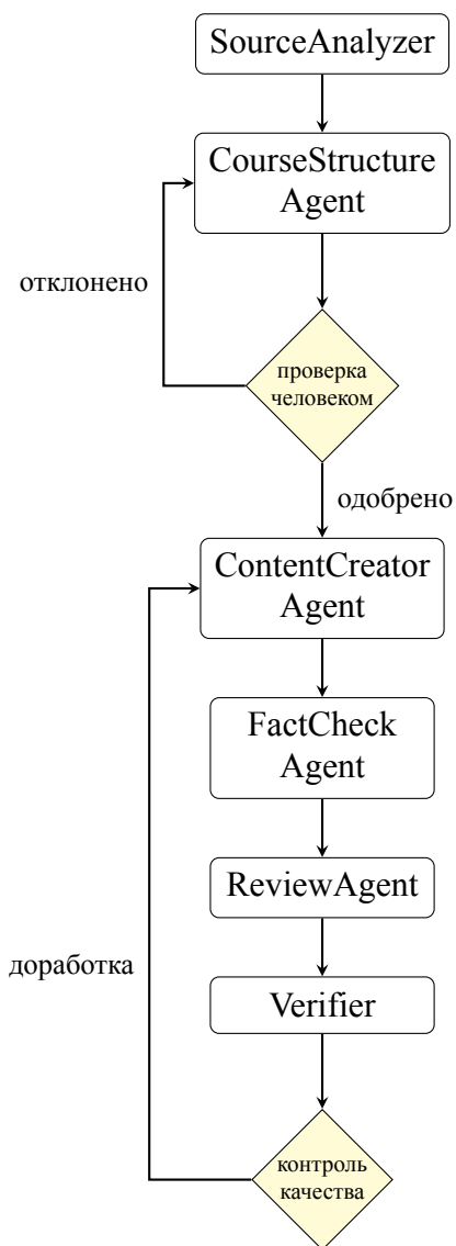
Рисунок 3.1 — Граф агентов ИИ-методиста (шестиузловой LangGraph StateGraph)
