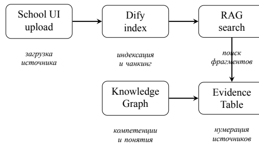
Рисунок 3.2 — Контур обработки источника и сборки EvidenceTable
