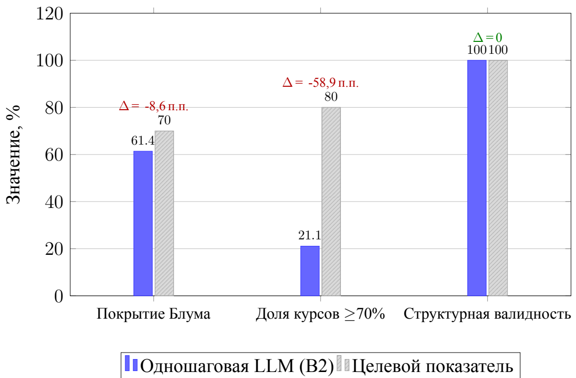
Рисунок 4.1 — Результаты одношаговой LLM-конфигурации (B2) и целевые показатели
