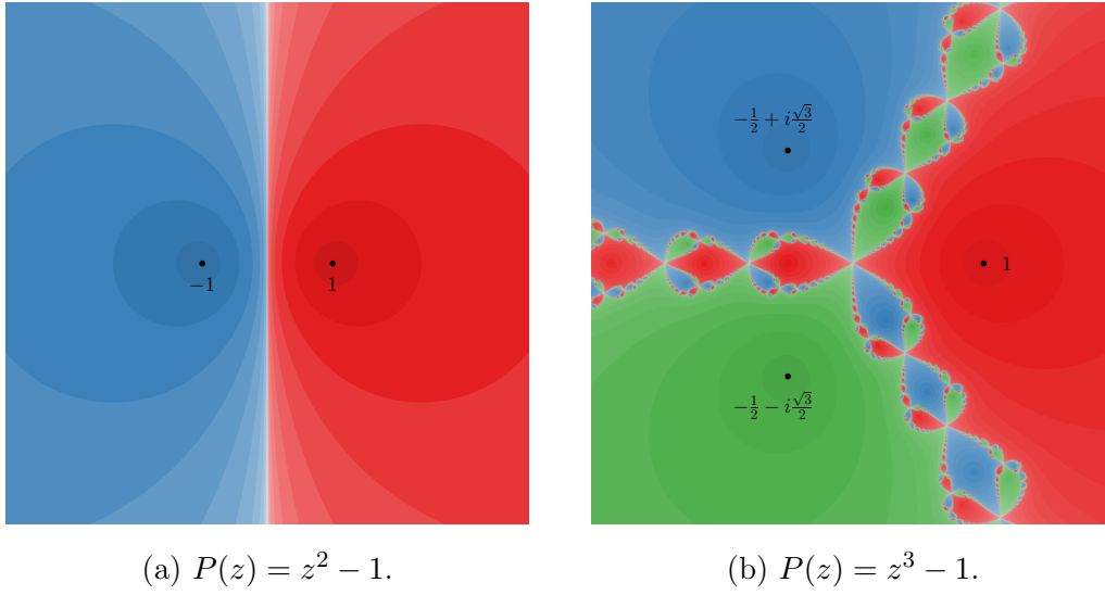
Figura 1.3: Planos dinámicos de N_P(z) . Cada color representa el conjunto de puntos que convergen a una misma raíz de P (cuantas más oscuros, mayor velocidad de convergencia).
