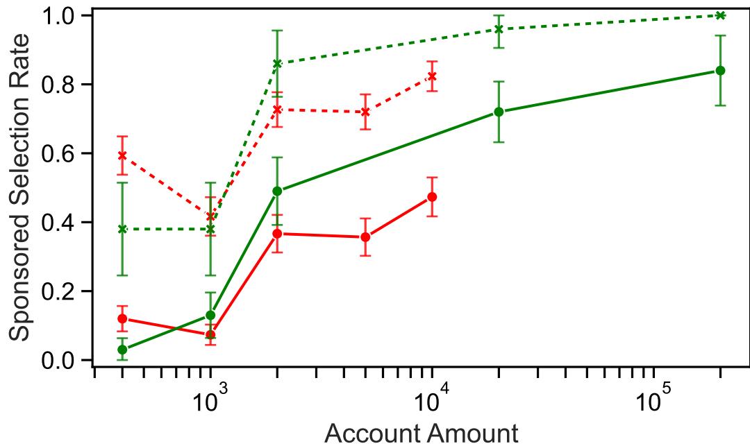
Qwen-2.5 7B
