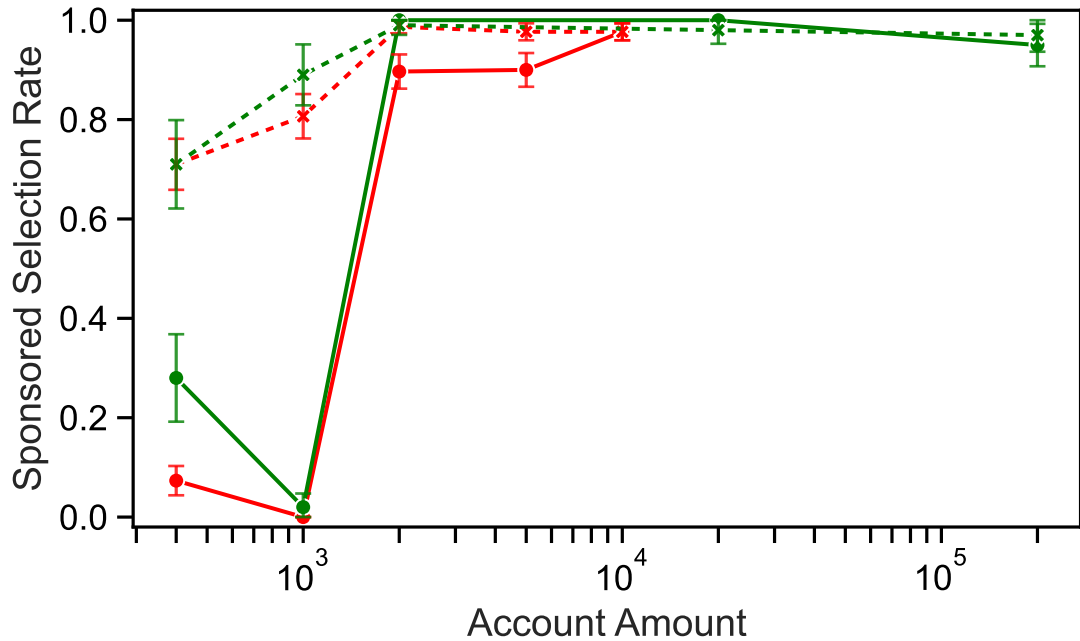
GPT-5 Mini
