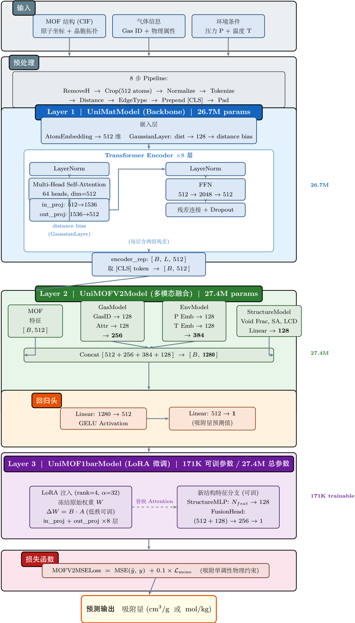
Uni-MOF 模型架构图
