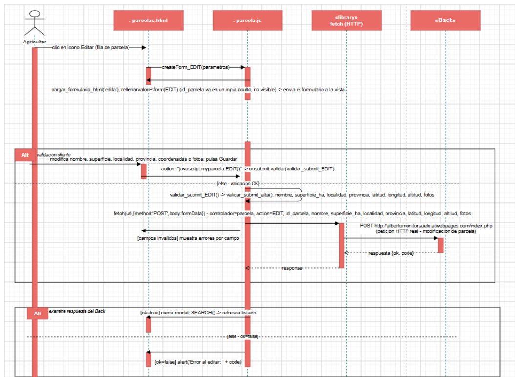
Figura II.10: Diagrama de secuencia detallado de Modificar Parcela
