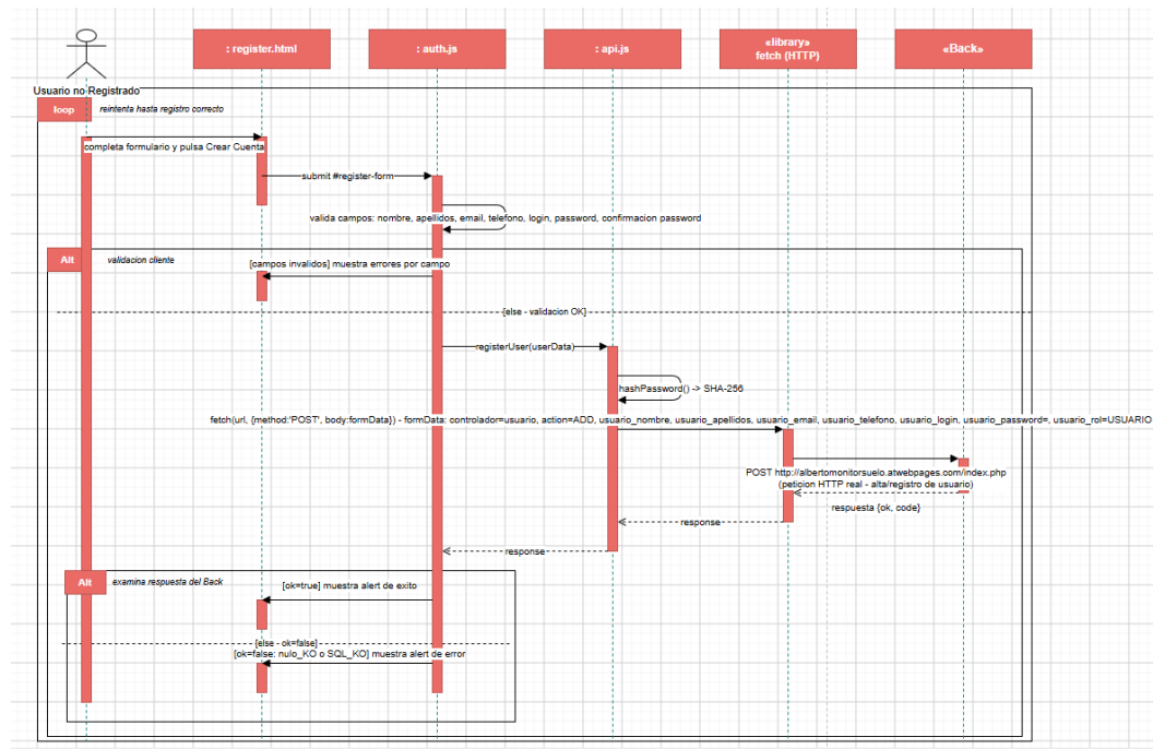
Figura II.3: Diagrama de secuencia detallado de Alta Usuario
