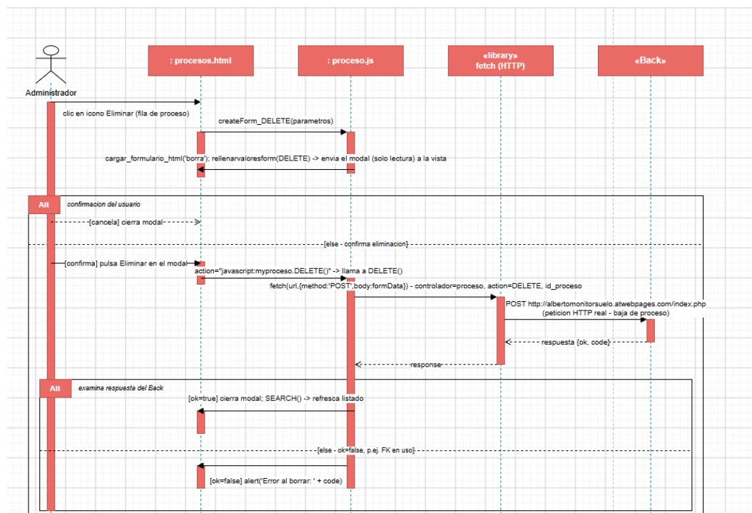
Figura II.21: Diagrama de secuencia detallado de Baja Proceso
