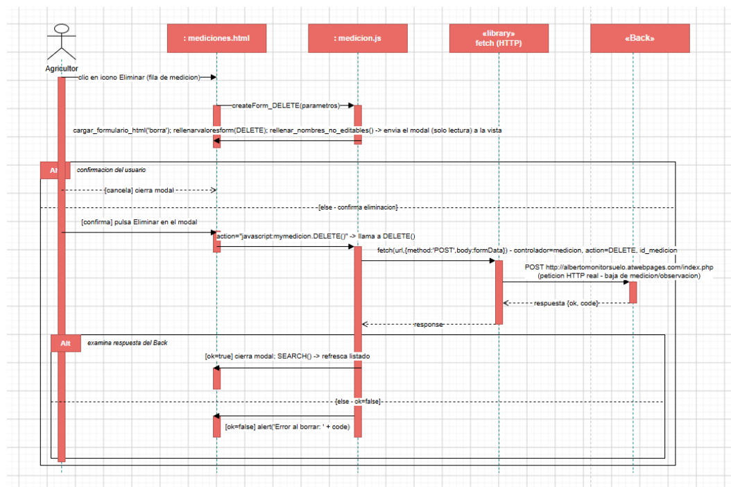
Figura II.16: Diagrama de secuencia detallado de Baja Medición
