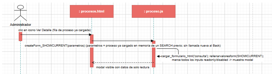
Figura II.19: Diagrama de secuencia detallado de Ver Detalle Proceso
