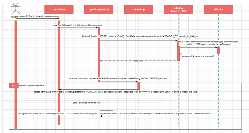
Figura II.4: Diagrama de secuencia detallado de Consultar Perfil
