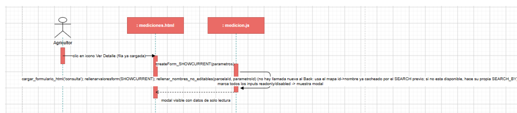
Figura II.14: Diagrama de secuencia detallado de Ver Detalle Medición
