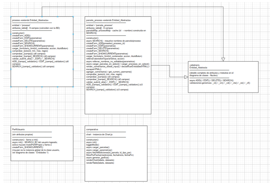
Figura 8.3: Diagrama de Clases segunda parte de las entidades
