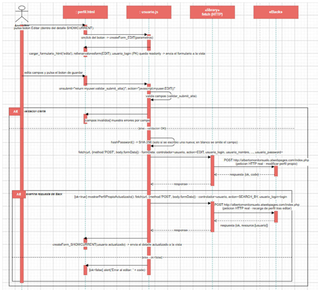
Figura II.5: Diagrama de secuencia detallado de Modificar Perfil
