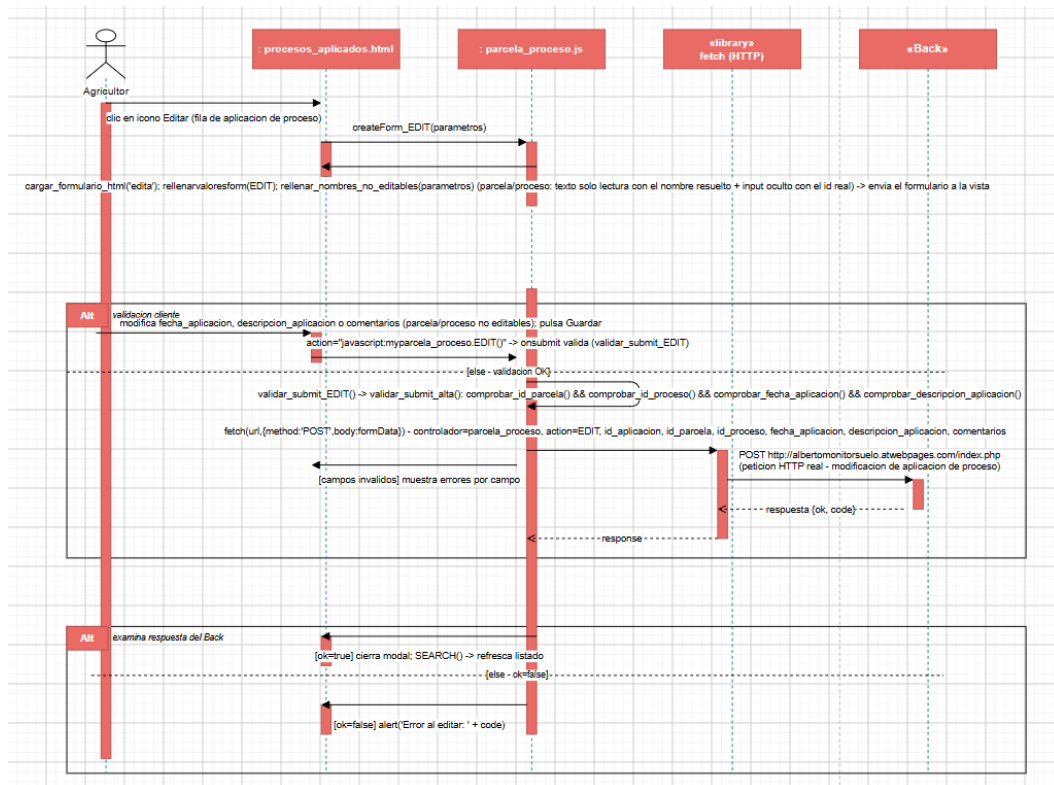
Figura II.25: Diagrama de secuencia detallado de Modificar Proceso Aplicado
