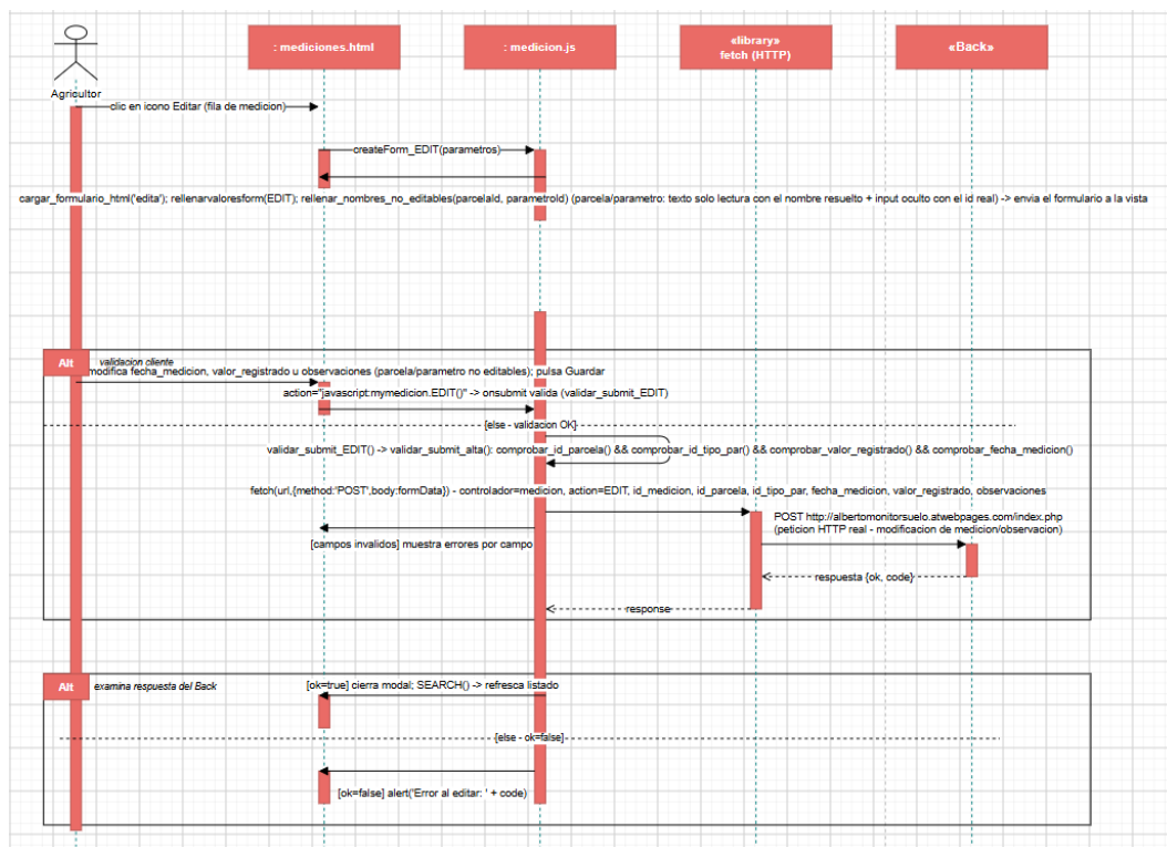
Figura II.15: Diagrama de secuencia detallado de Modificar Medición
