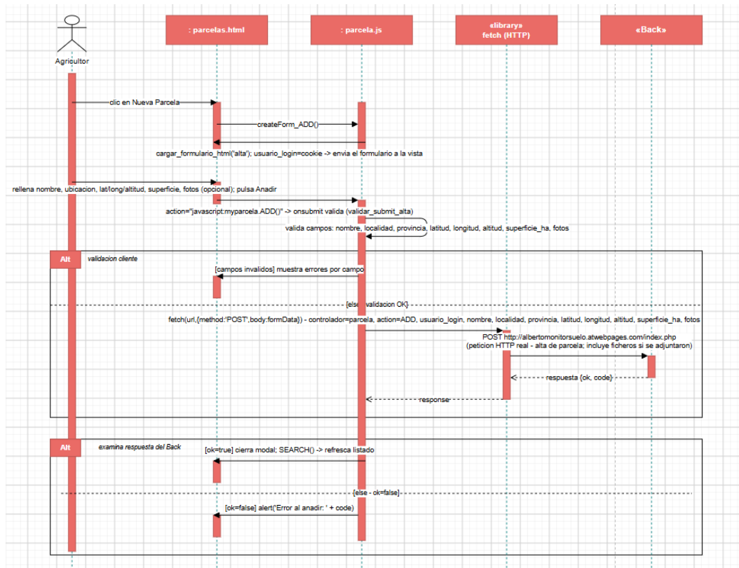
Figura II.7: Diagrama de secuencia detallado de Alta Parcela
