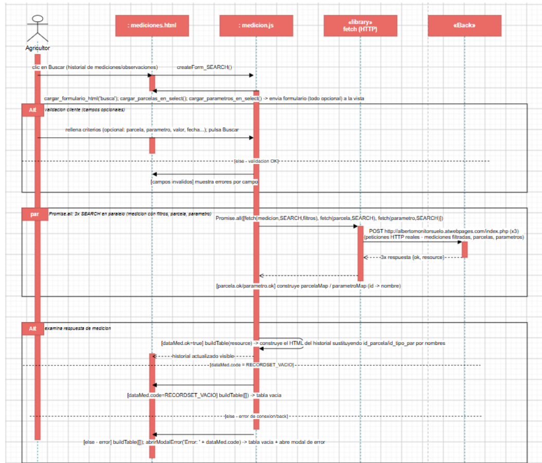
Figura II.13: Diagrama de secuencia detallado de Consultar Historial Mediciones
