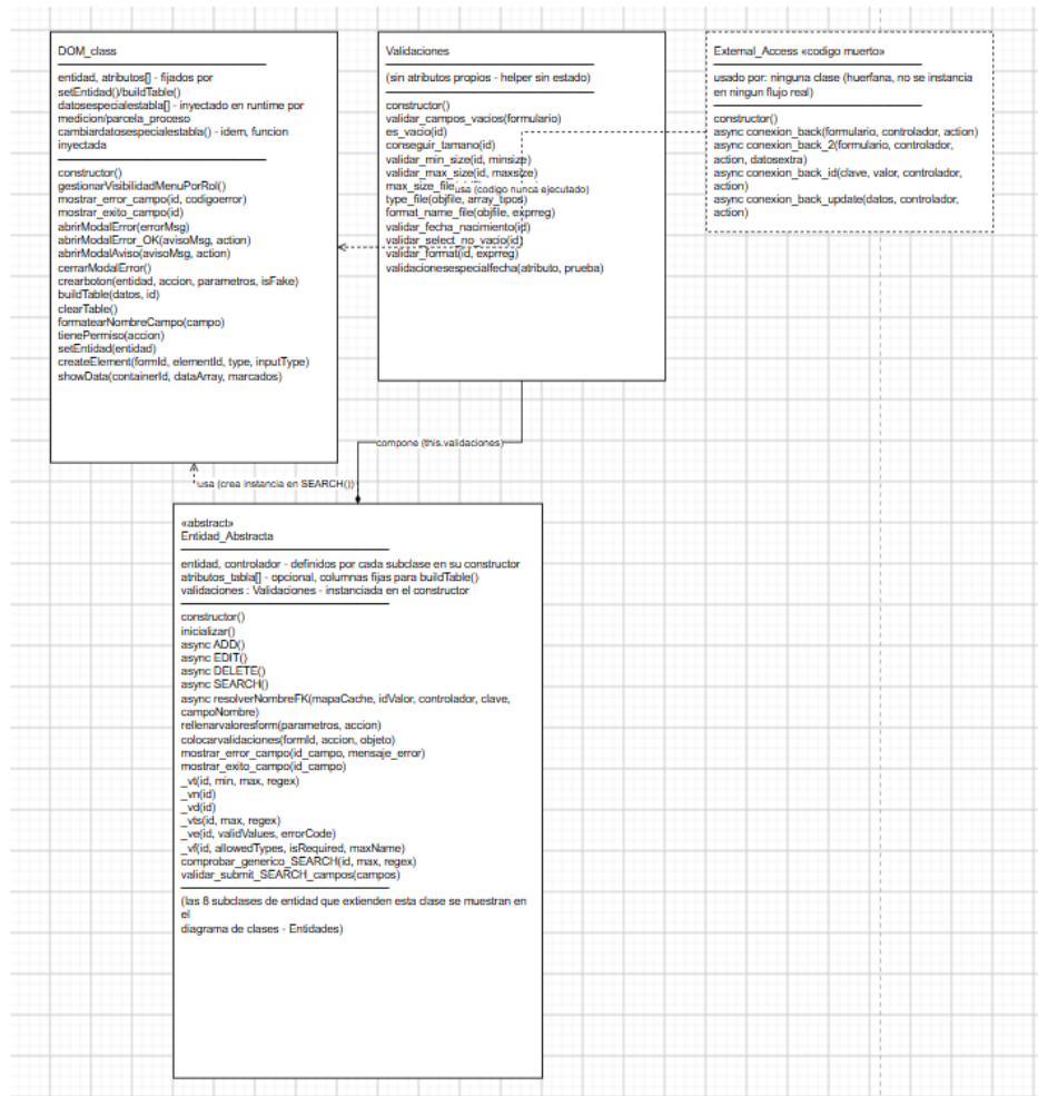
Figura 8.1: Diagrama de Clases núcleo
