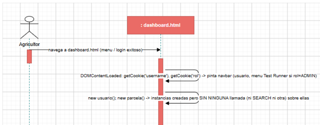
Figura II.27: Diagrama de secuencia detallado de Visualizar Dashboard
