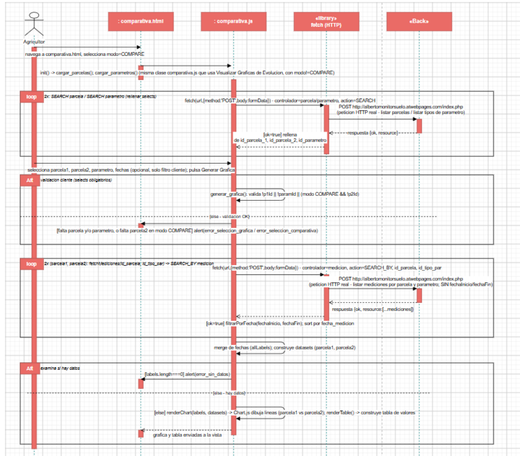
Figura II.29: Diagrama de secuencia detallado de Comparar Resultados
