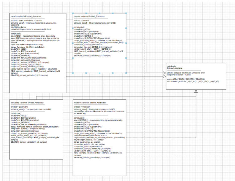
Figura 8.2: Diagrama de Clases primera parte de las entidades
