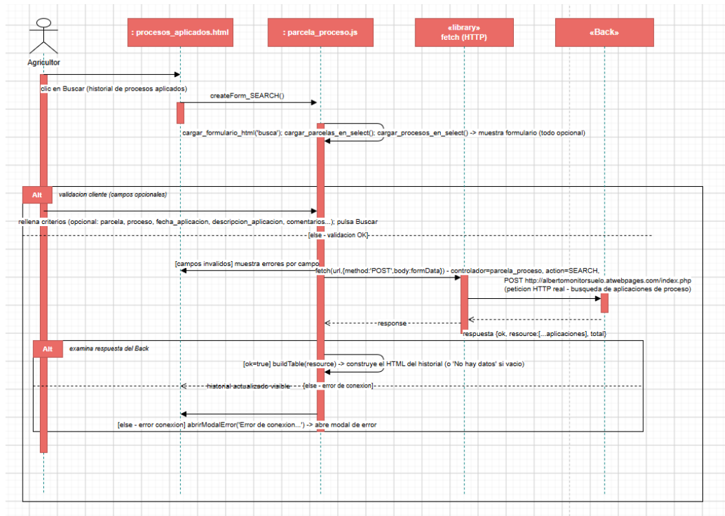
Figura II.23: Diagrama de secuencia detallado de Consultar Historial Procesos
