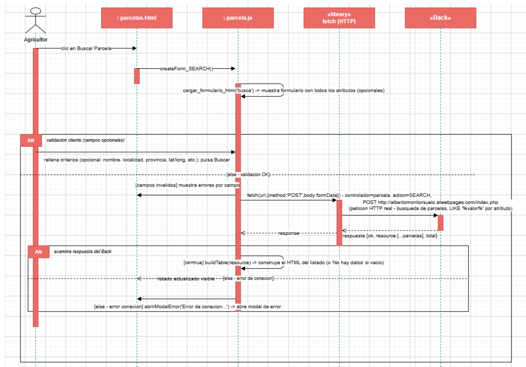
Figura II.8: Diagrama de secuencia detallado de Consultar Parcelas
