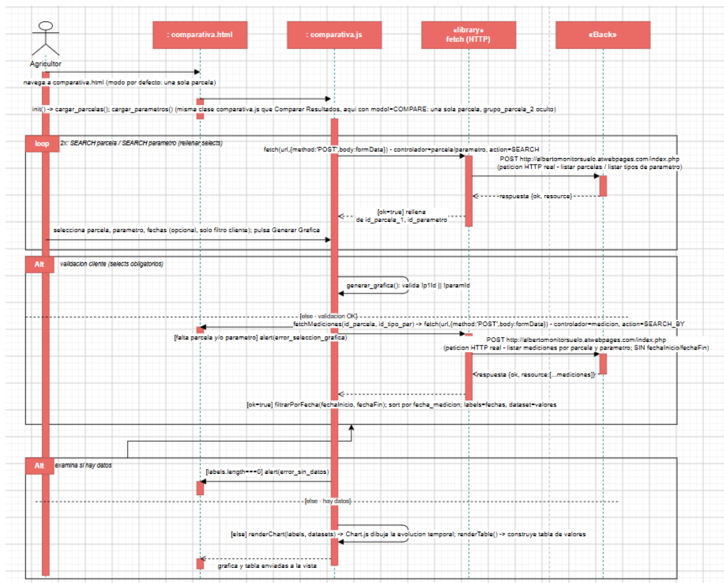
Figura II.28: Diagrama de secuencia detallado de Visualizar Gráficas Evolución
