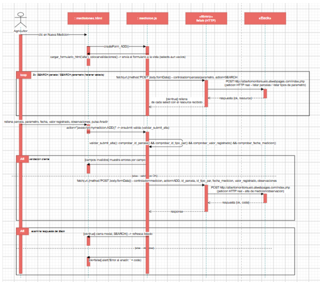
Figura II.12: Diagrama de secuencia detallado de Alta Medición
