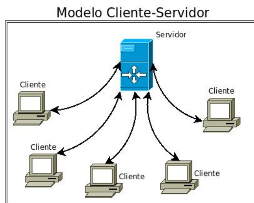
Figura 3.1: Arquitectura Cliente-Servidor
