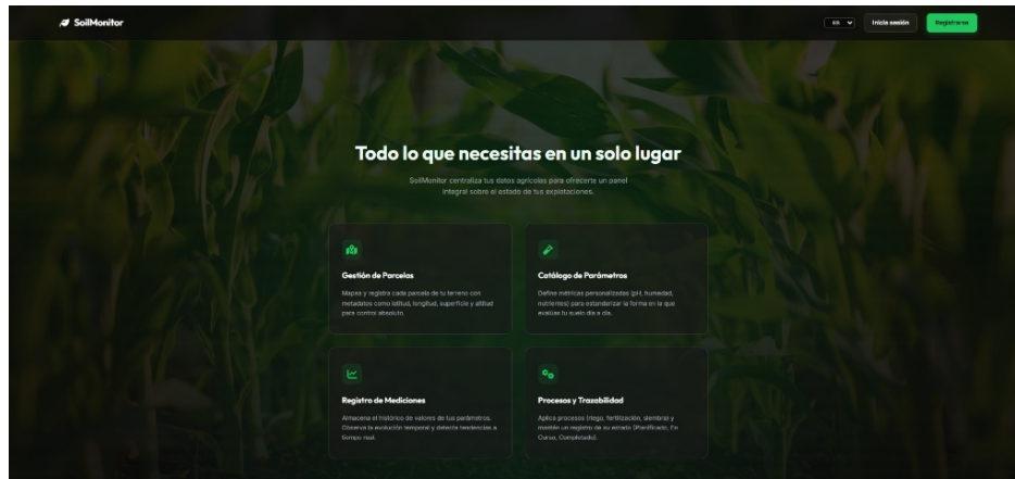
Figura 8.6: Pantalla inicial
