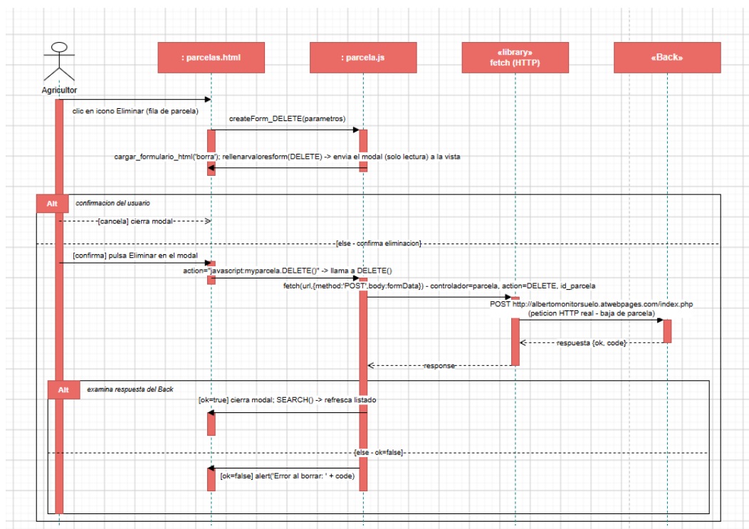
Figura II.11: Diagrama de secuencia detallado de Baja Parcela
