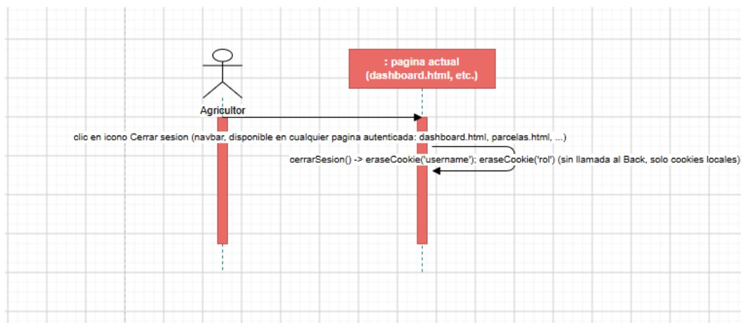
Figura II.1: Diagrama de secuencia detallado de Cerrar Sesión
