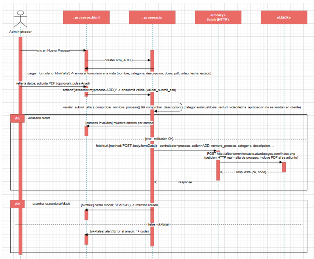
Figura II.17: Diagrama de secuencia detallado de Alta Proceso
