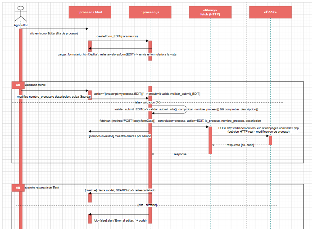
Figura II.20: Diagrama de secuencia detallado de Modificar Proceso
