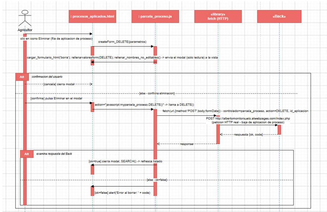
Figura II.26: Diagrama de secuencia detallado de Baja Proceso Aplicado
