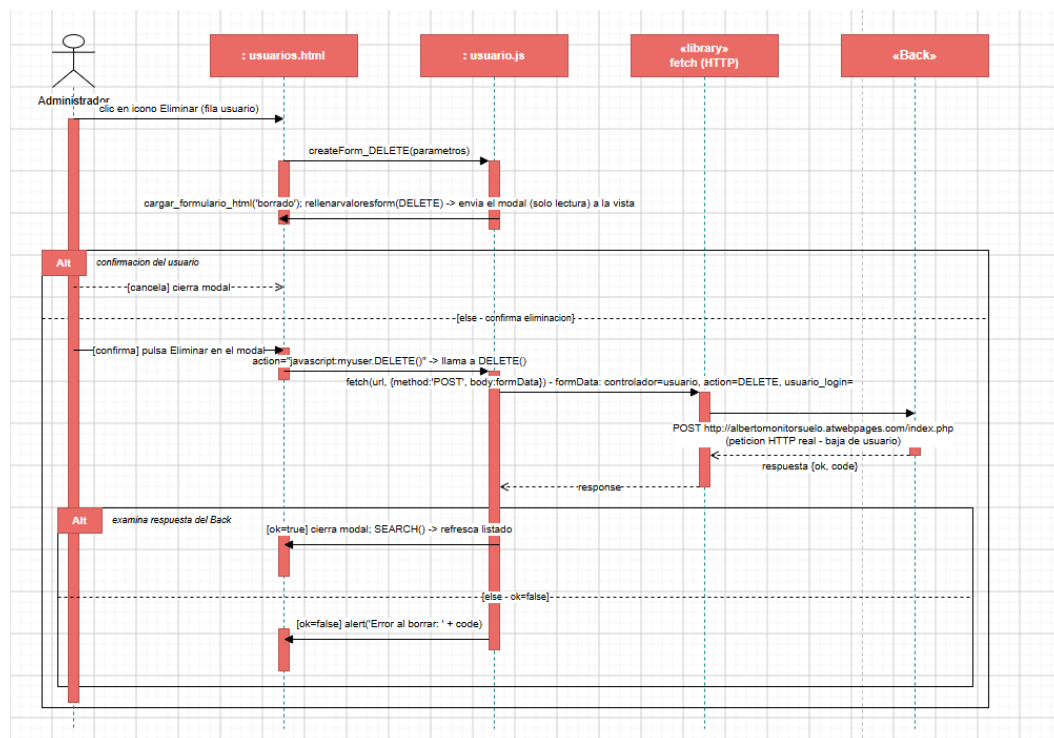
Figura II.6: Diagrama de secuencia detallado de Baja Usuario
