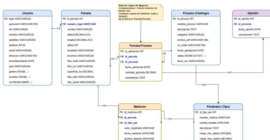
Figura 9.1: Diagrama Entidad-Relación
