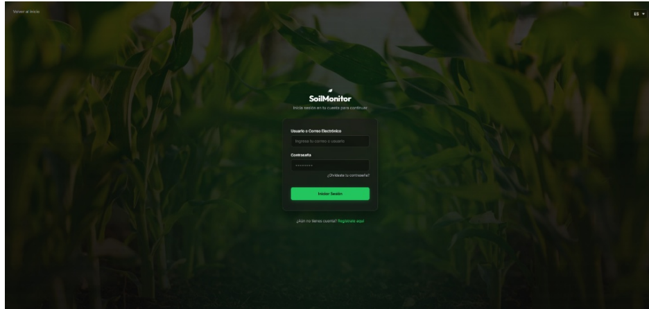
Figura 8.8: Login
