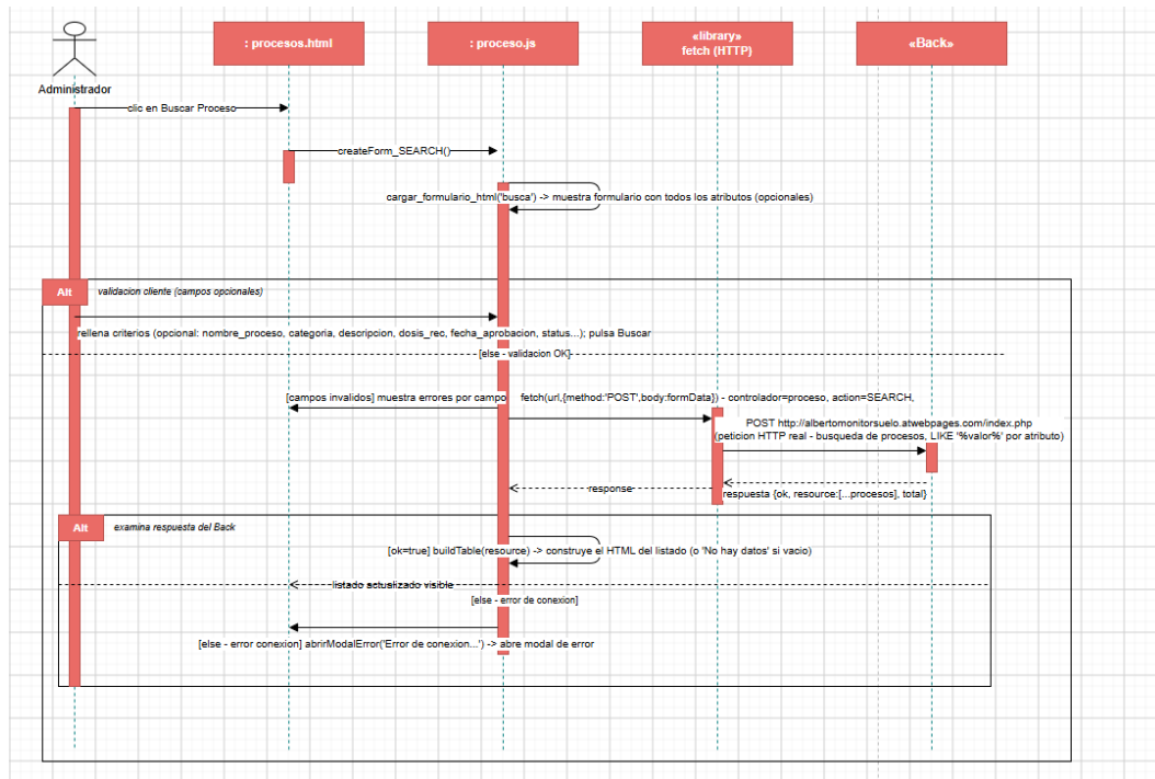
Figura II.18: Diagrama de secuencia detallado de Consultar Proceso
