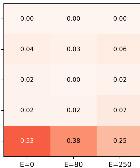
Llama 3.3 70B
