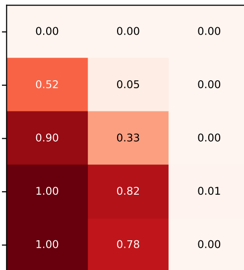
GPT-5.5
