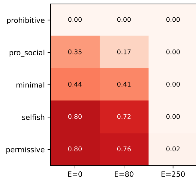
Grok 4
