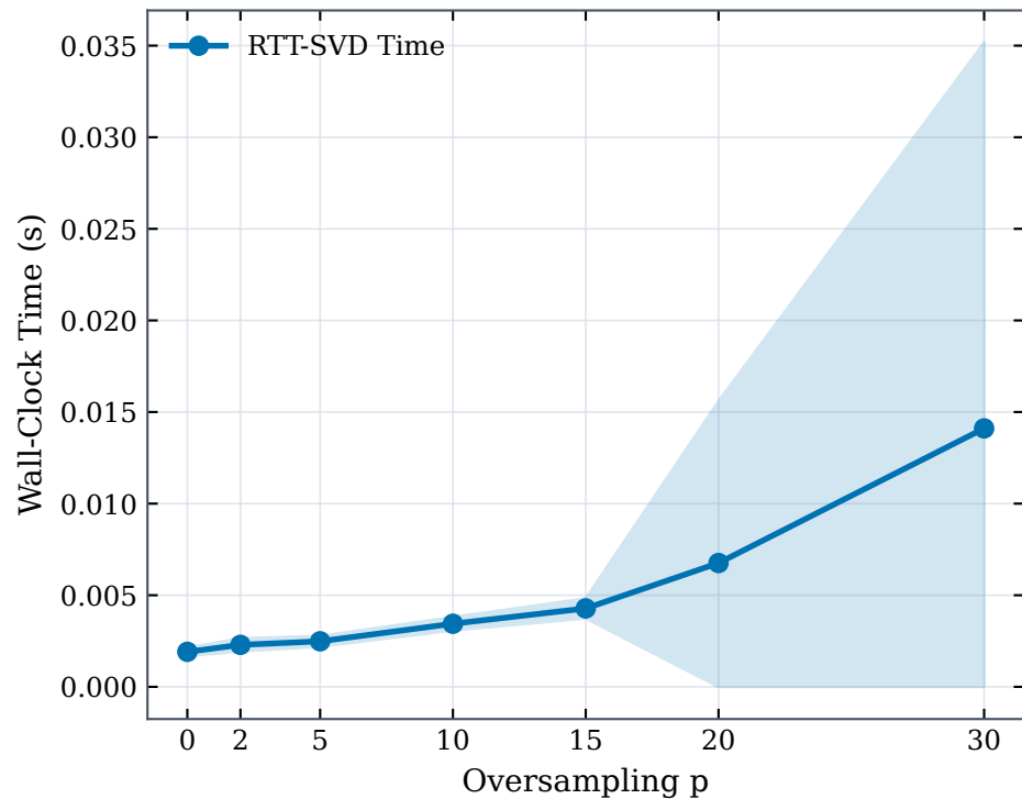
Computation Time vs Oversampling Parameter
