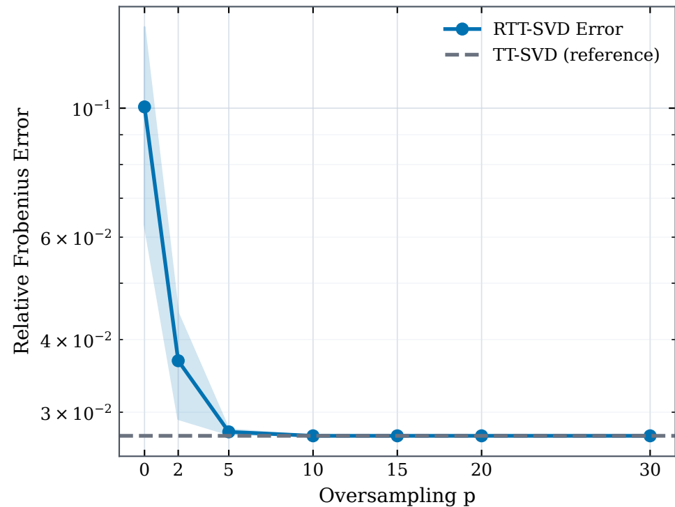
Error vs Oversampling Parameter
