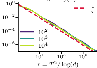
T \gg \log(d)
