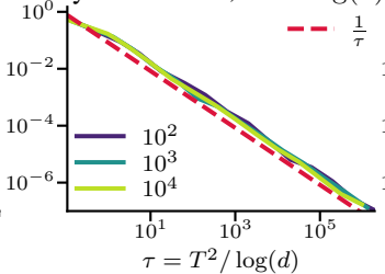
Synthetic Data, T \gg \log(d)
