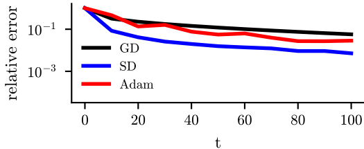
Quadratic (MSE)
