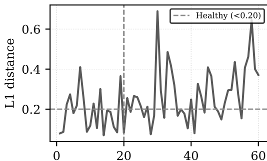
(d) Train-val load L1
