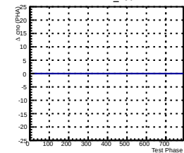
TREND1_230
