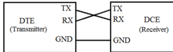
Fig: RS-232
