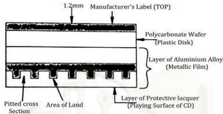
Fig: Layout CD-ROM Disc
