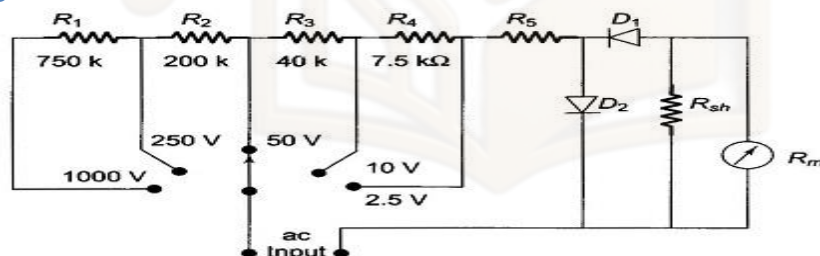
Fig: multirange ac voltmeter
