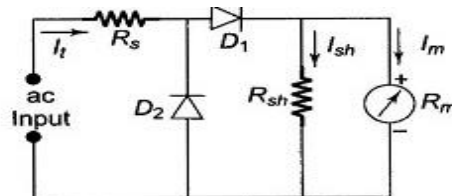
Fig: General rectifier type ac voltmeter
