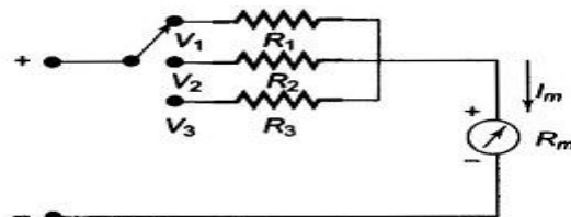
Fig. 4.2 Multirange Voltmeter
