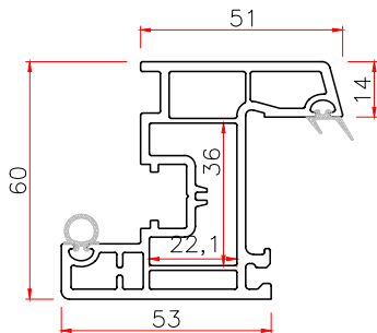
60 INWARD SASH
