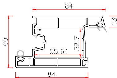
60T INWARD DOOR SASH Code: P60NMS-T THK WT 2.2 1.61
