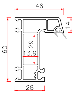
6046 CASEMENT FRAME
