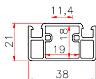
SCREEN SASH MULLION Code: TSSZT THK WT 1.7 0.39
