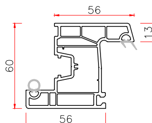
60T INWARD SASH Code: P60NS-T THK WT 2.2 1.30
