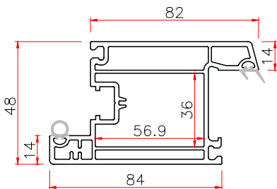
60 INWARD DOOR SASH
