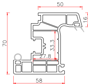
70 INWARD SASH
