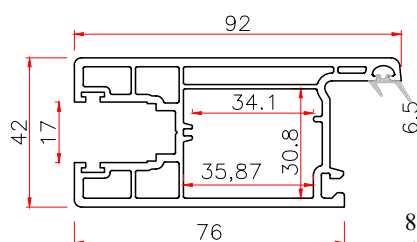
8886 DOOR SASH
