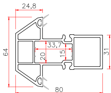
80 MULLION Code: T80ZT THK WT 2.2 1.22
