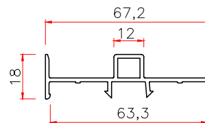
120 INTERLOCK
